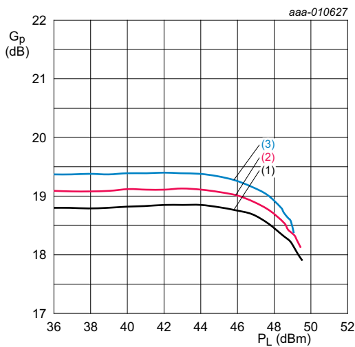
V_{DS} = 28\text{ V}; I_{Dq} = 1300\text{ mA} . (1) f = 2305\text{ MHz} (2) f = 2350\text{ MHz} (3) f = 2395\text{ MHz}
