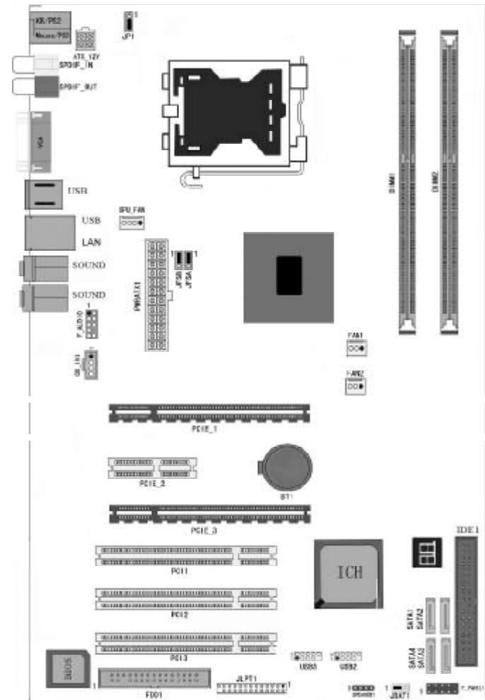
C. G946- MVP Ver2.0 主机板布局图
