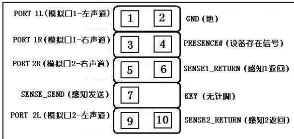
AC97 与 HD 音频连接座引脚定义对比表
