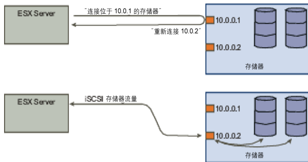
图 1-6. 端口重定向
