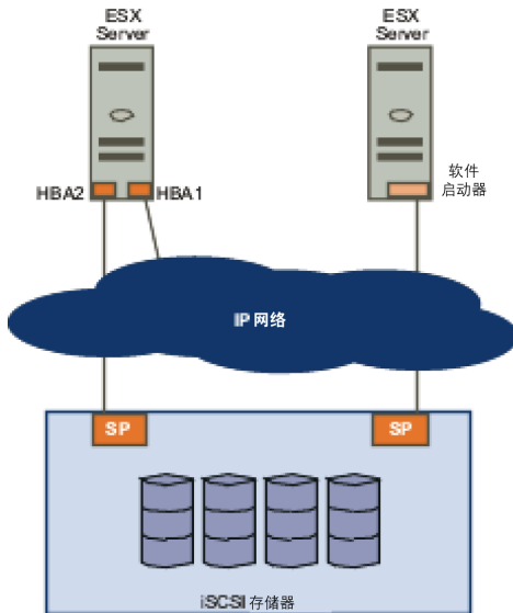
图 1-5. 多路径和故障切换
