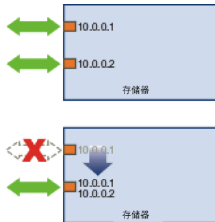
图 1-7. 端口重新分配
