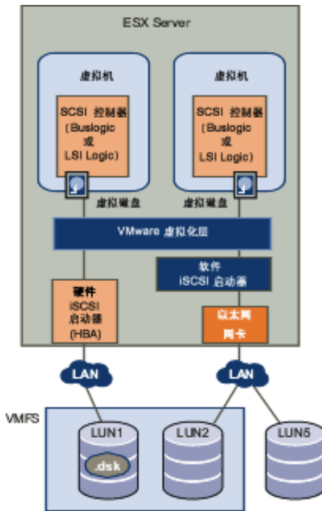
图 1-1. iSCSI SAN 存储虚拟化
