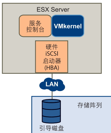
图 4-1. 从 SAN 引导如何运作
