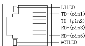
CN30: 网络接口
