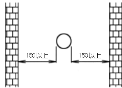
给排气管出口正面
