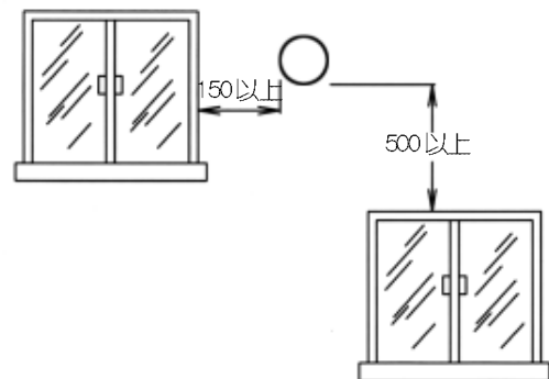
给排气管出口距进风口距离
