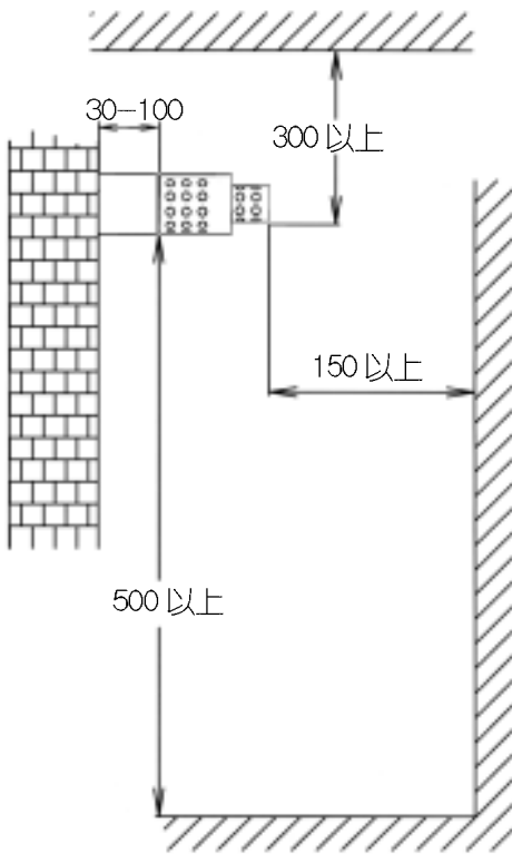
给排气管出口侧面
